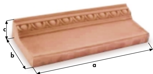
cornice a ovuli
