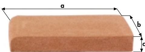
mattone smussato
