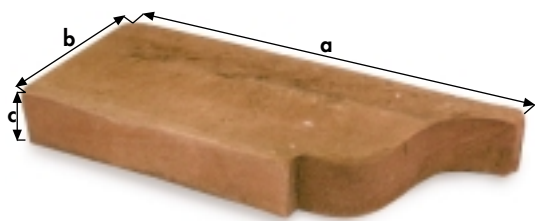
cornice verticale di gronda
