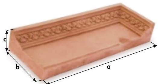
angolo cornice foglie
